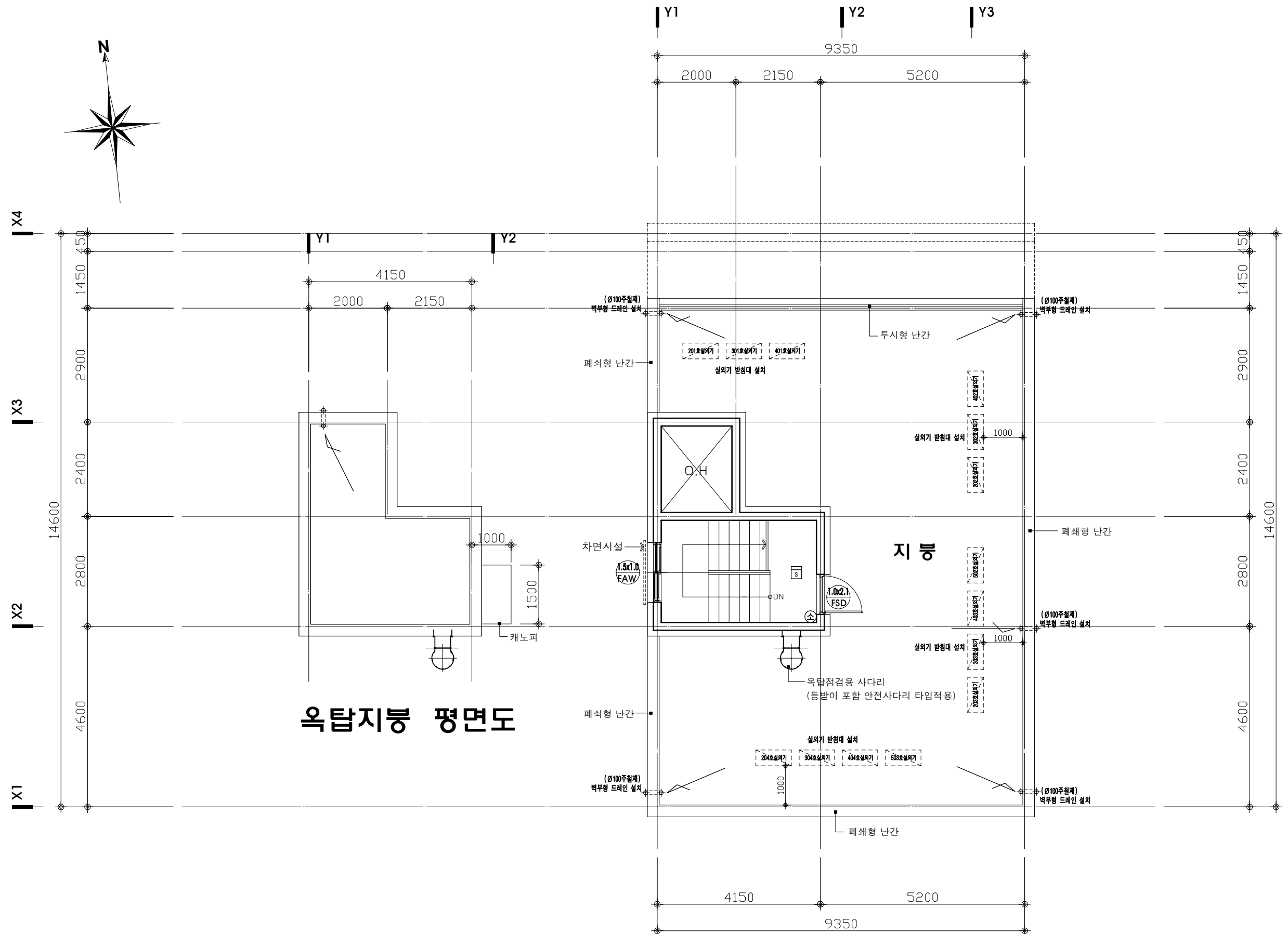
지붕 및 옥탑층 평면도 SCALE : 1/100
