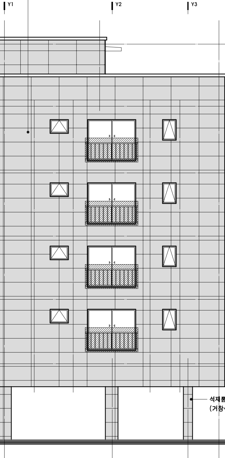
배 면 도 (남측) SCALE : 1/100
