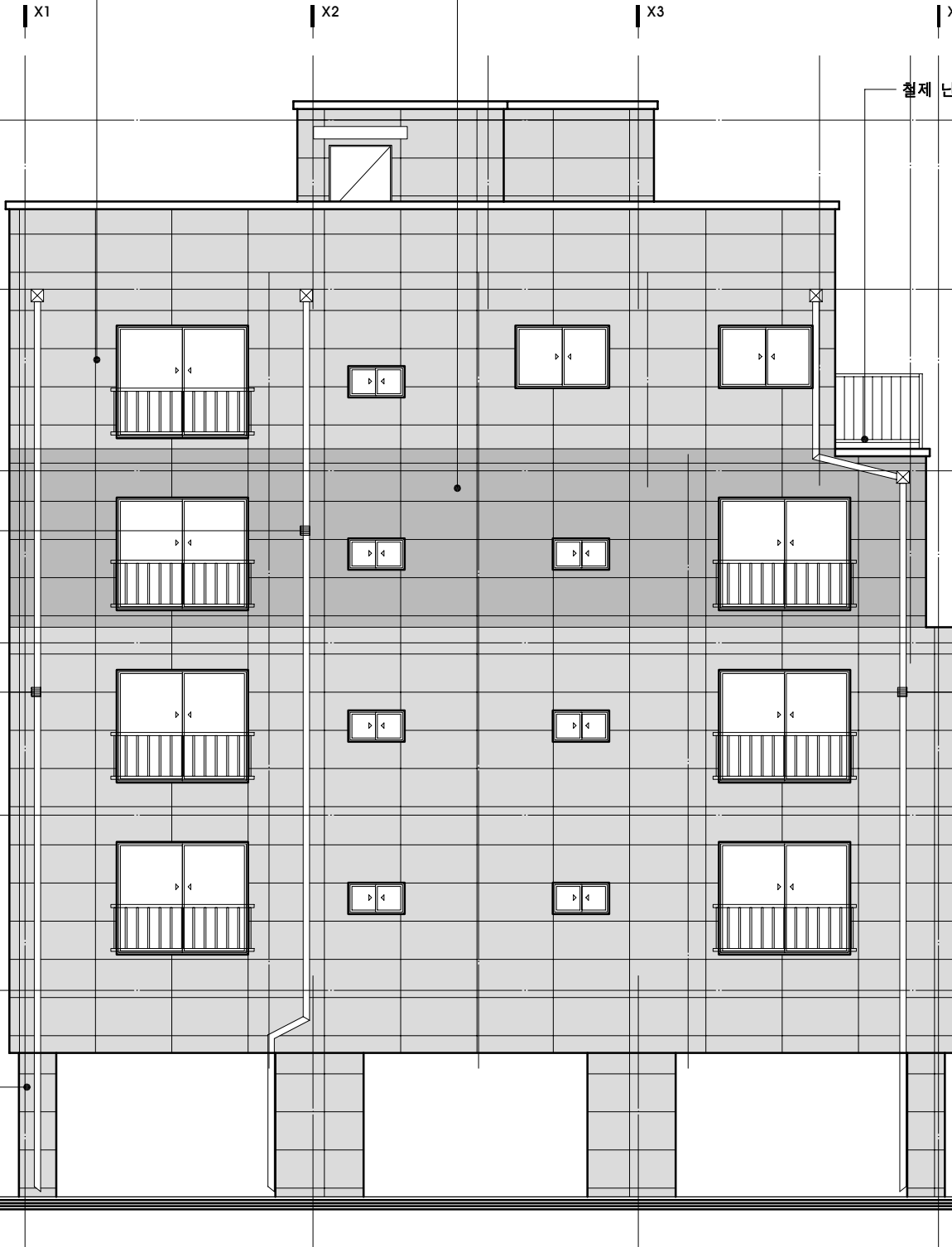
좌 측 면 도 (동측) SCALE : 1/100
