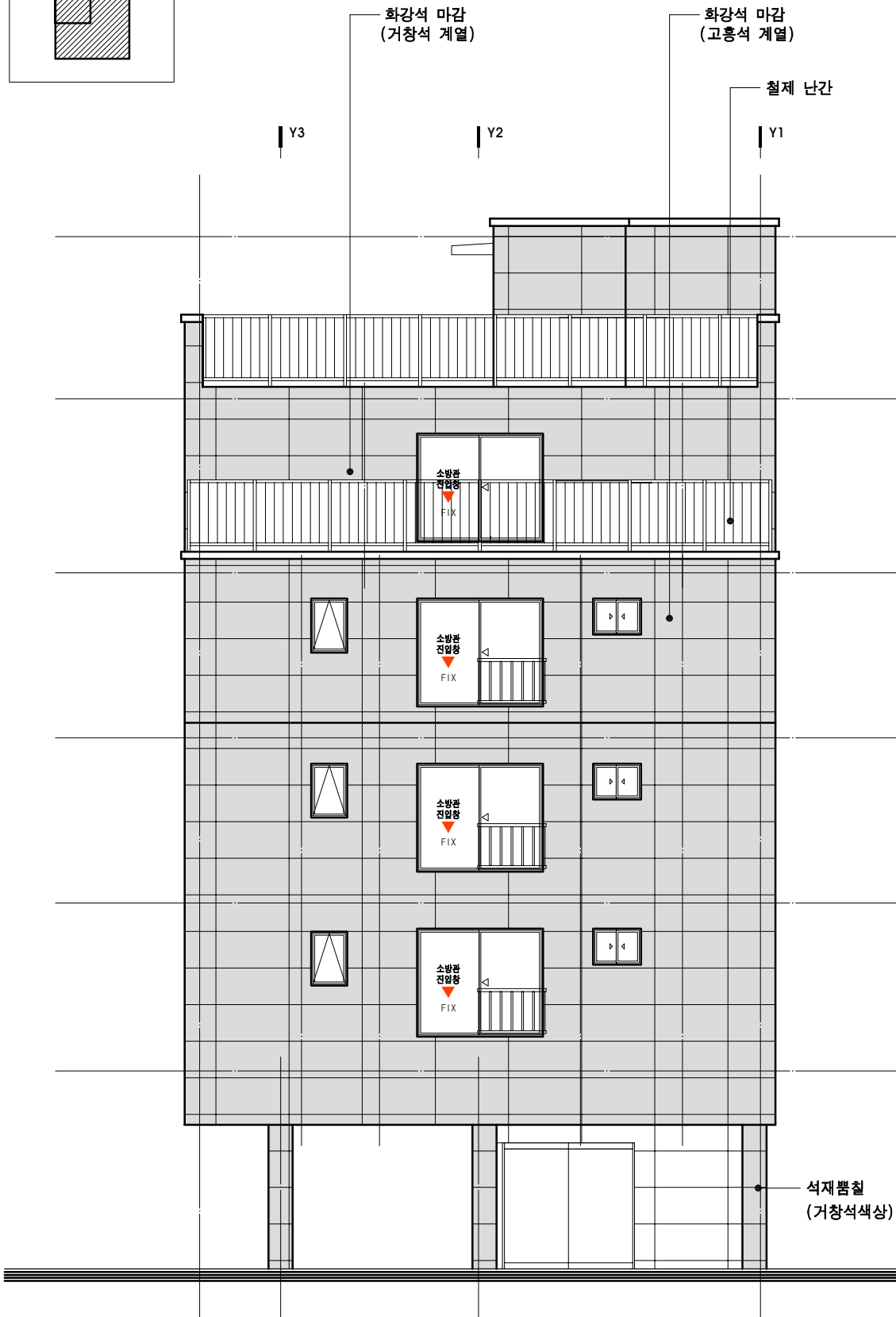
정면도 (북측) SCALE : 1/100
