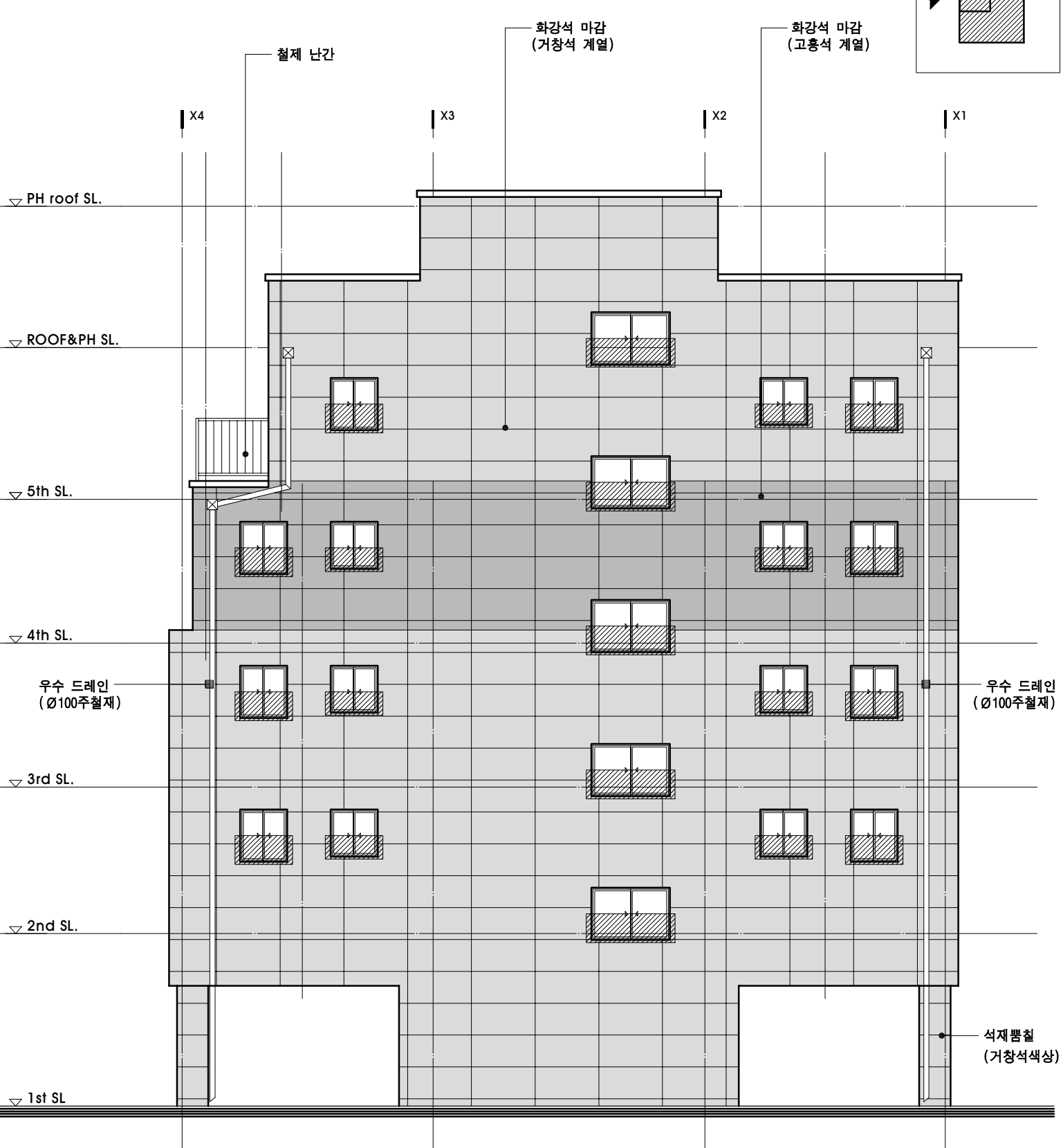
우측면도 (서측) SCALE : 1/100
